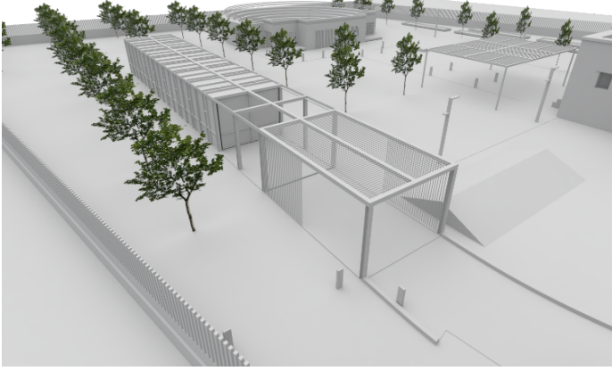
Κατασκευή υπαίθριου θερμοκηπίου, πρόπλασμα
