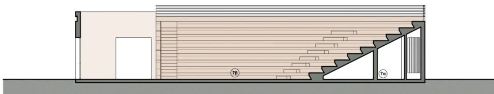
Κατασκευή υπαίθριου θεάτρου, Πρόσοψη & Τομή
