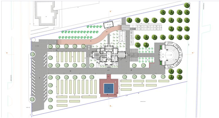
Οριζοντιογραφία Α
