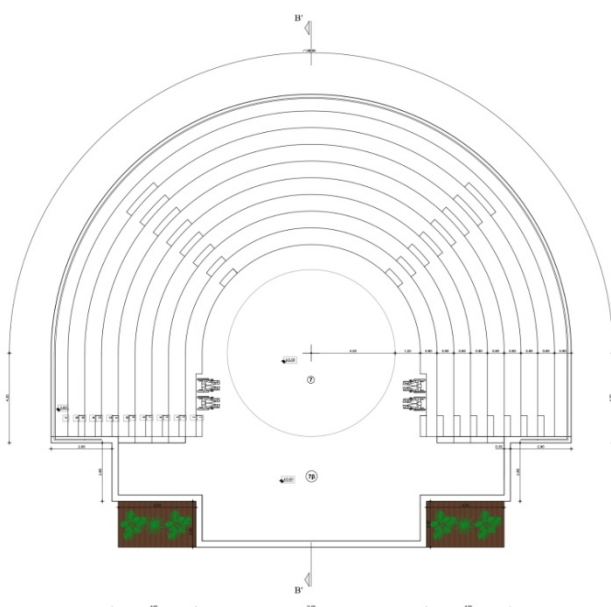
Κατασκευή υπαίθριου θεάτρου, Κατοψεις
